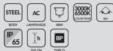
KAREN 2 RO-P4086
